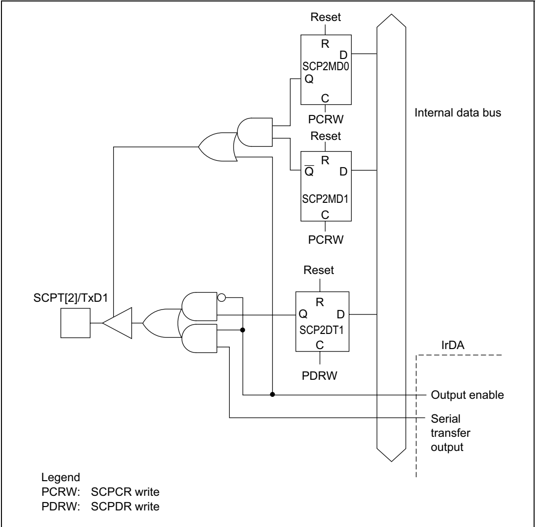
Figure 18.3 SCPT[2]/TxD1 Pin
